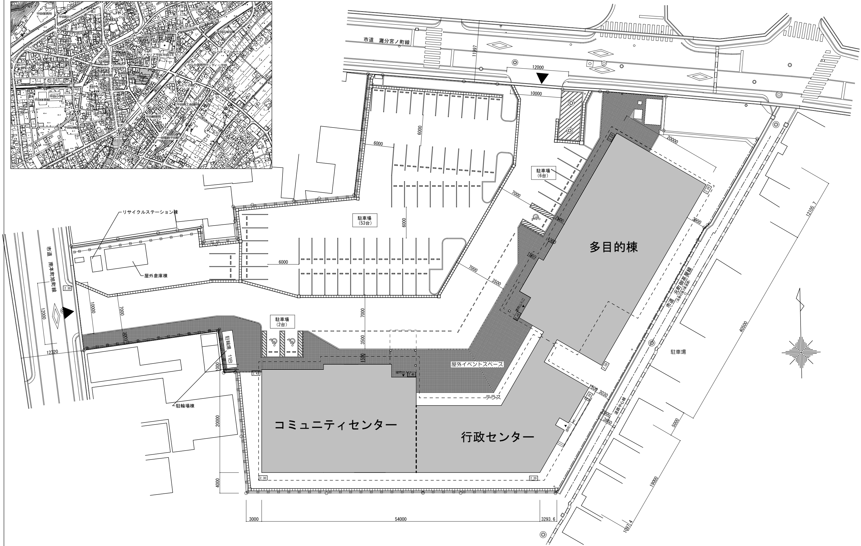
配置図
