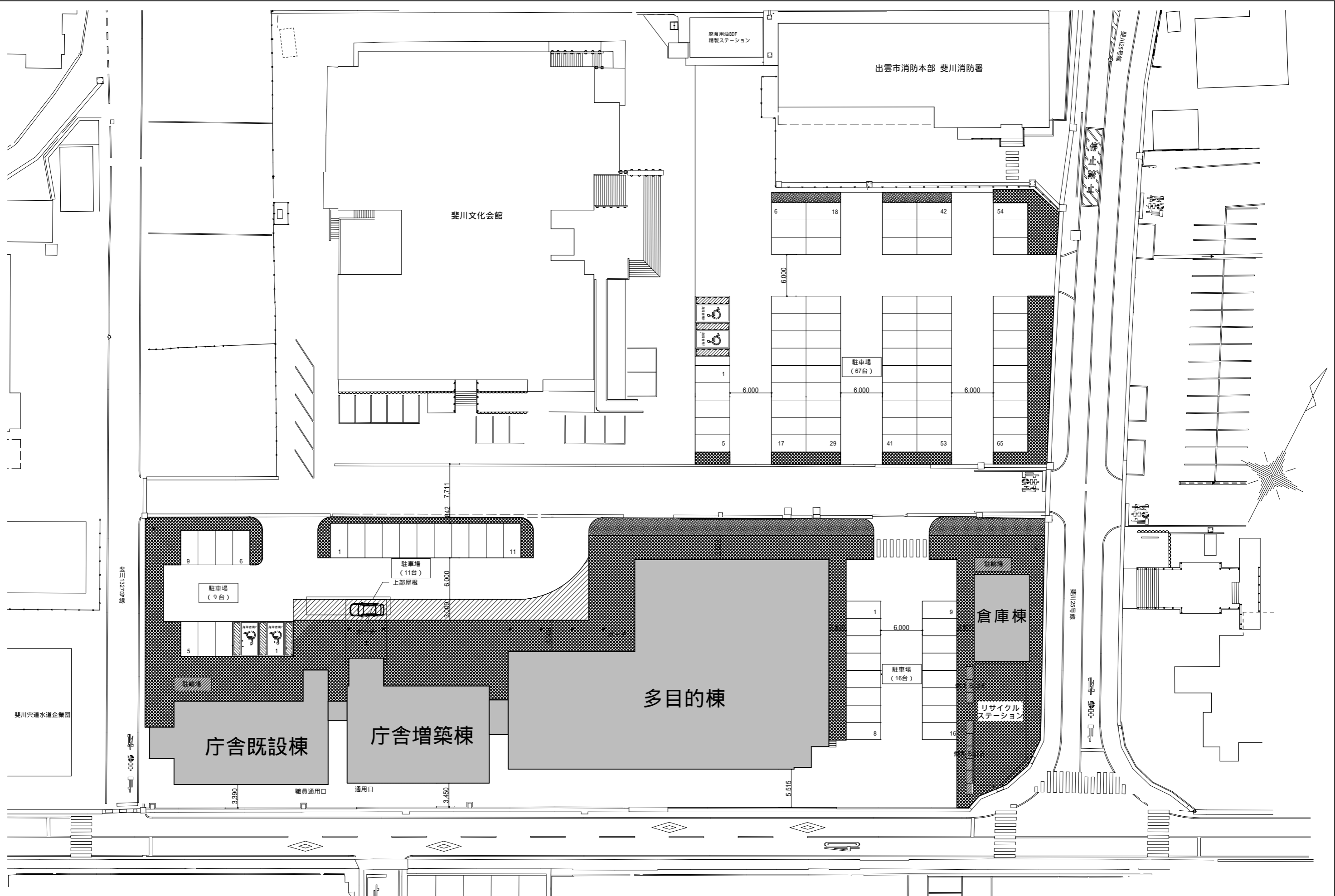
配置図
