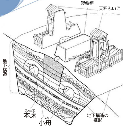
たたら製鉄炉と地下構造の模式図
