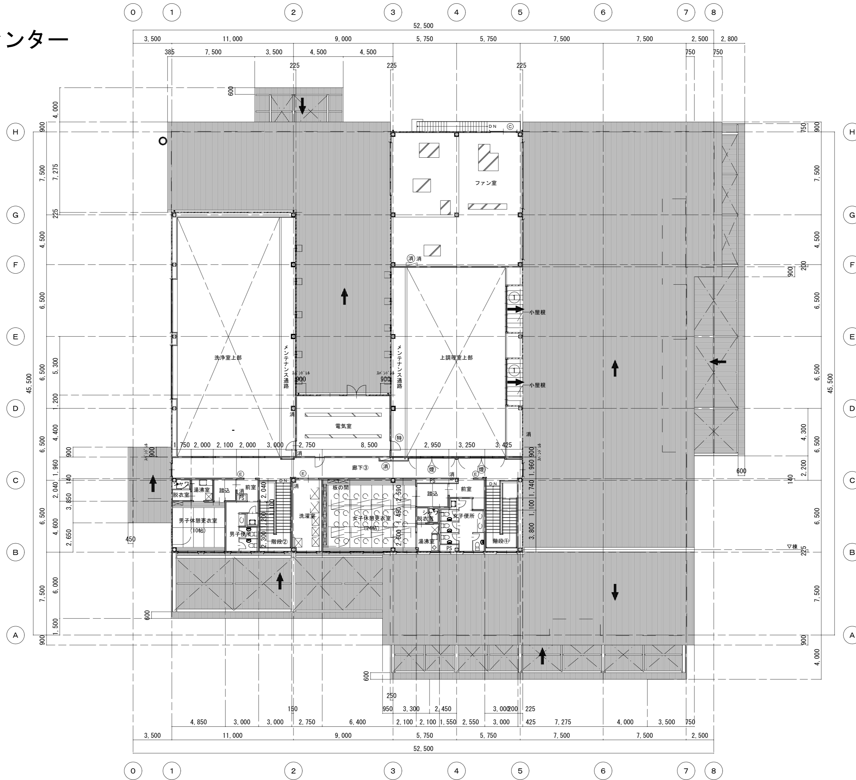
2階平面図 1 : 200 (A2)
