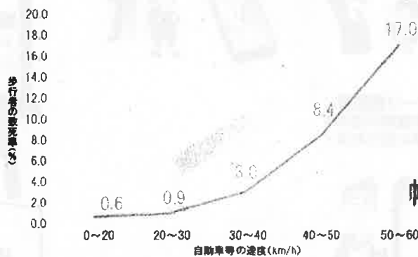
自動車等の速度と歩行者の致死率
