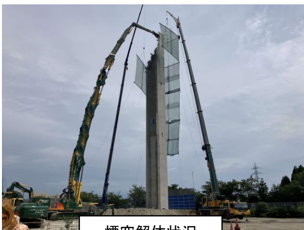
煙突解体状況
