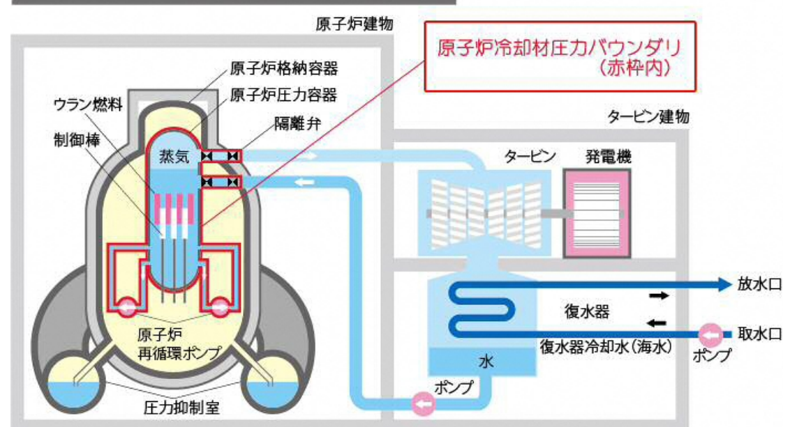
原子炉冷却材圧力バウンダリの範囲（イメージ）
